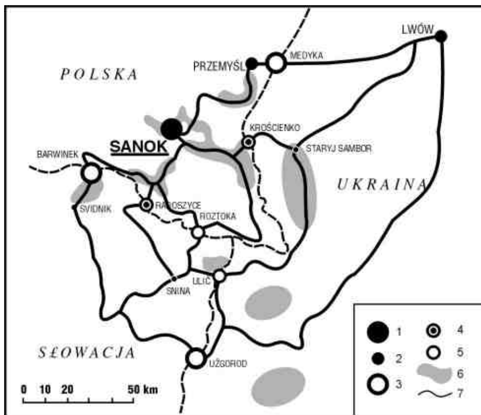
Ryc 1. Szlak ikon w Euroregionie Karpackim 1 - główny punkt węzłowy szlaku, 2 - inne punkty węzłowe, 3 - istniejące drogowe przejścia graniczne, 4 - projektowane drogowe przejścia graniczne, 5 - pożądane przejścia graniczne, 6 - skupienia zabytkowych cerkwi (wstępna informacja o ukraińskich), 7 - proponowane warianty przebiegu szlaku.
